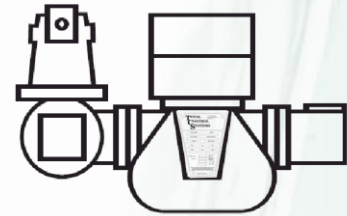
Syaç ,Gösterge, Hava Ayırıcı ,Filtre, Preset Numaratörü ve Preset Valfi
